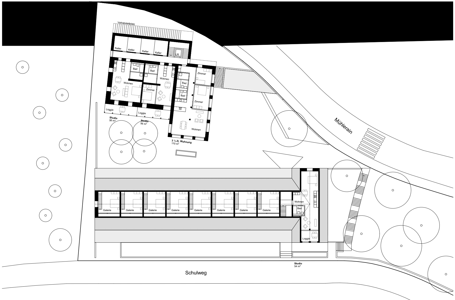
Aarfähre | Biberstein | Grundriss | Ebene 4
